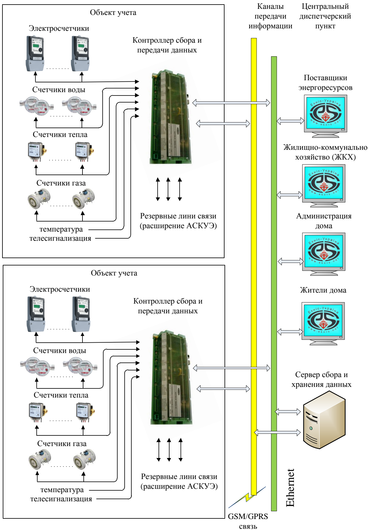
Структурная схема АСКУЭ ЖКХ
